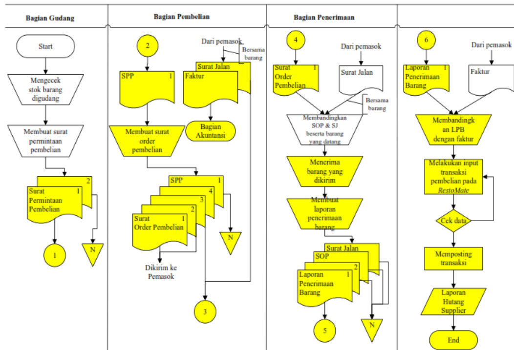
Gambar 3 Usulan Bagan Alir Dokumen Sistem Pembelian Kredit
