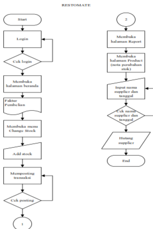
Gambar 2 Bagan Alir Pembelian Kredit Menggunakan Software RestoMate
